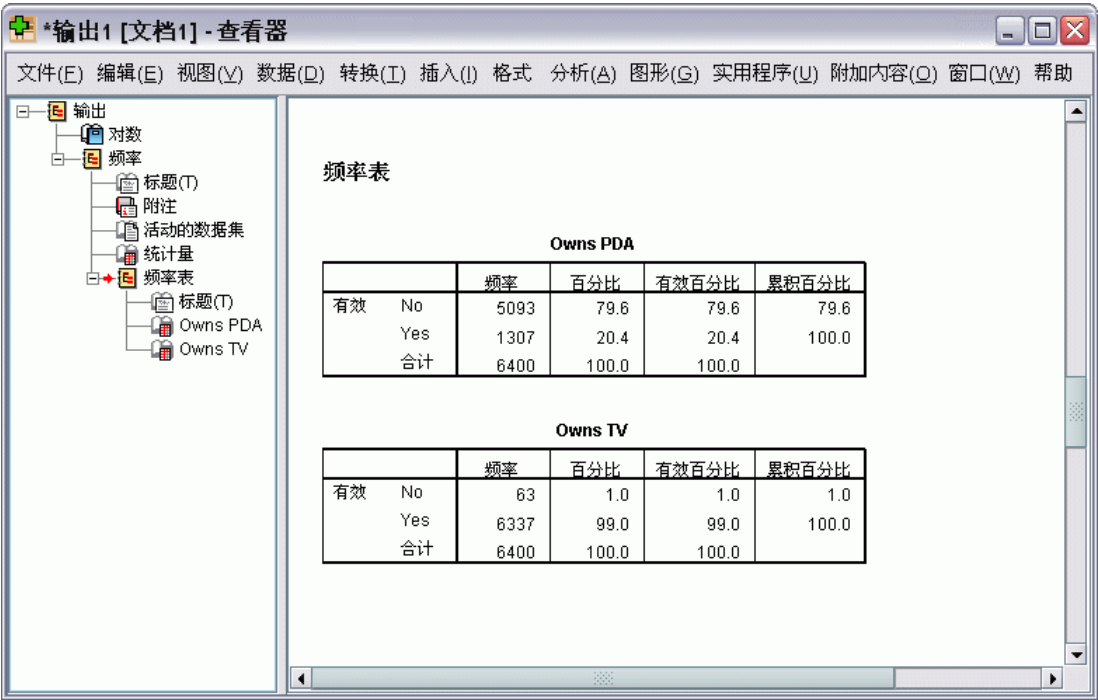
图片 5-2 频率表
