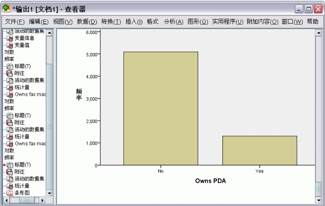
图片 5-5 条形图
