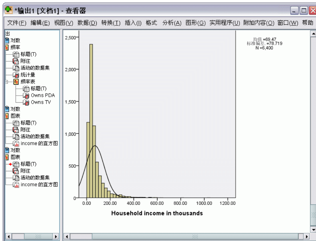
图片 5-10 直方图
