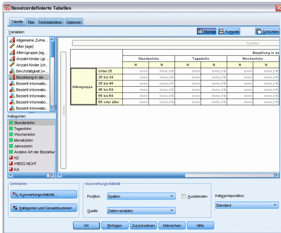
Abbildung 13-6 Tabellenvorschau mit geänderten Beschriftungen für Auswertungsstatistiken
