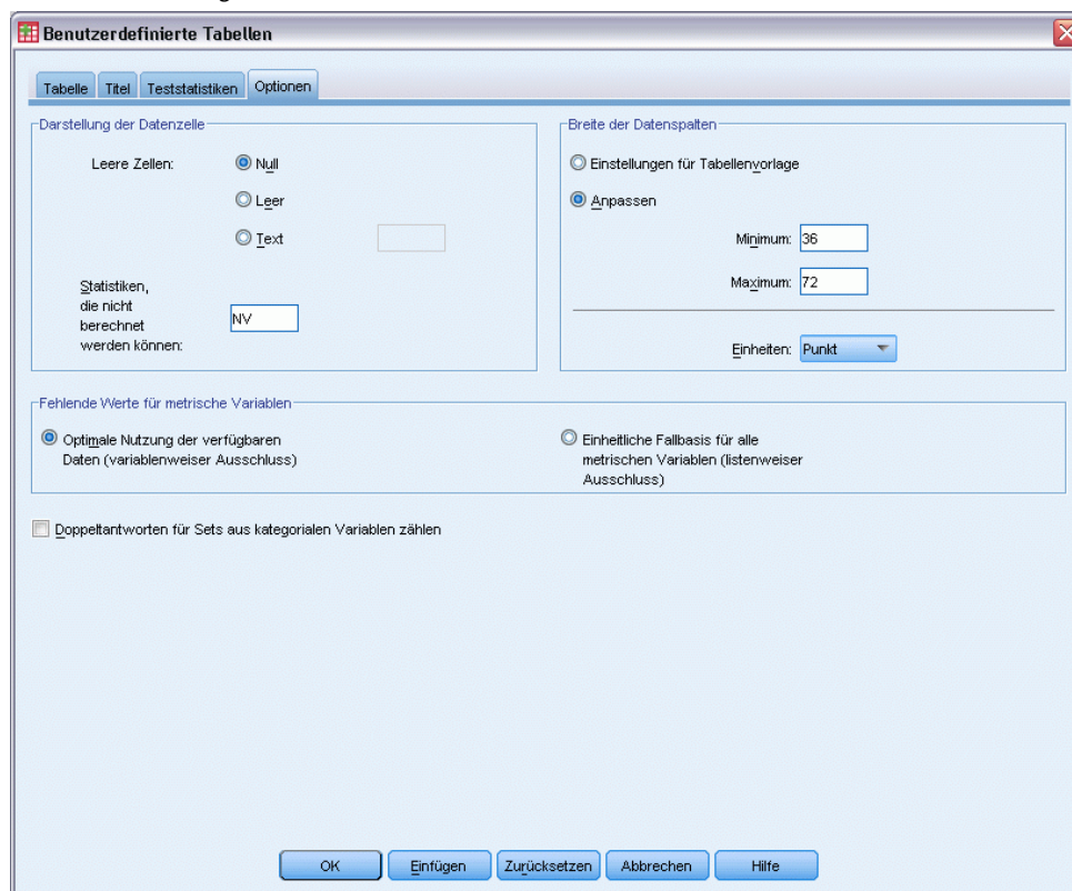
Abbildung 13-12 Ändern des Anzeigewerts für Statistiken, die nicht berechnet werden können
