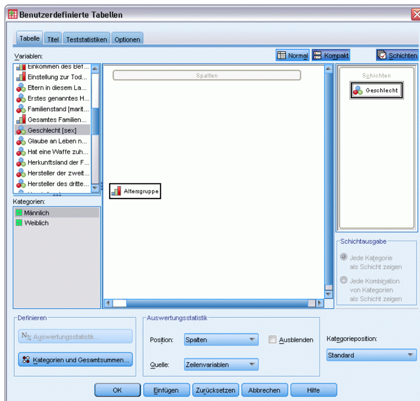
Abbildung 4-15 Alterskategorie in Zeilen, Geschlecht in Schichten
