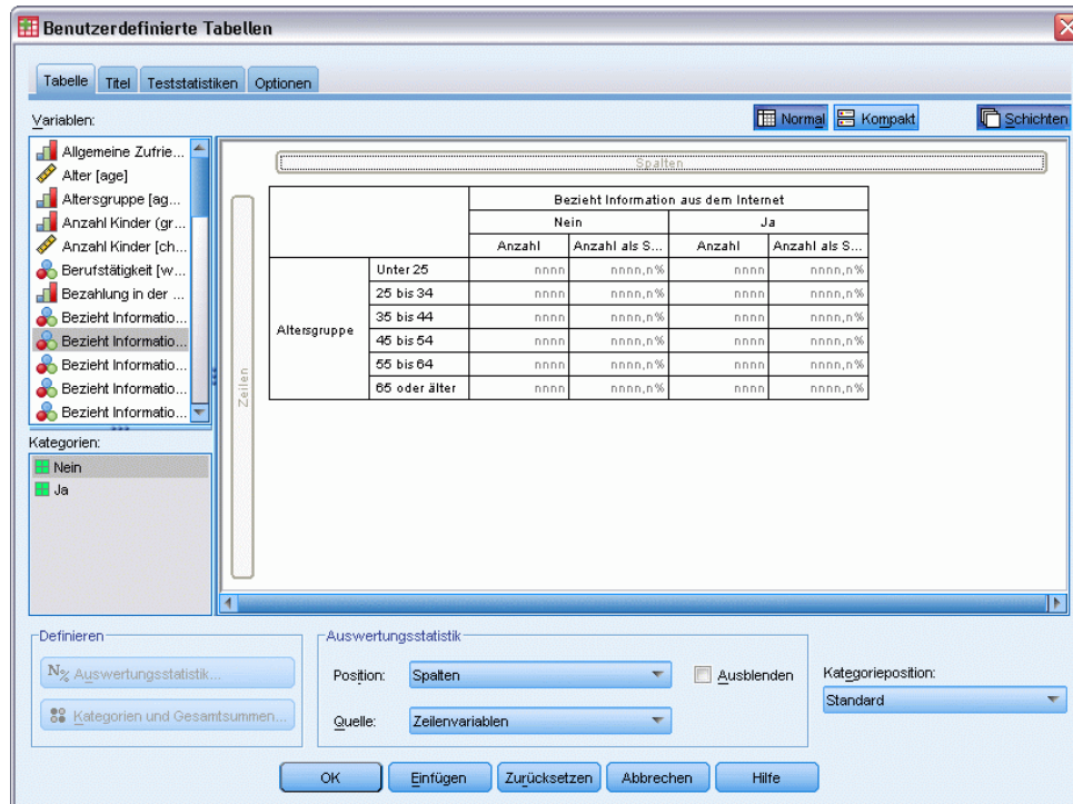
Abbildung 8-3 Kategoriale Variablen in Kreuztabellen
